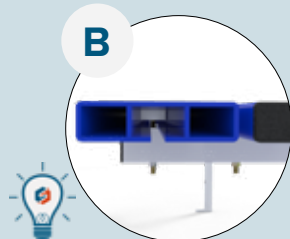
B Les lisses sont fixées à la structure grâce à des éclisses placées dans le rail interne afin de ne pas avoir de vis apparentes.
